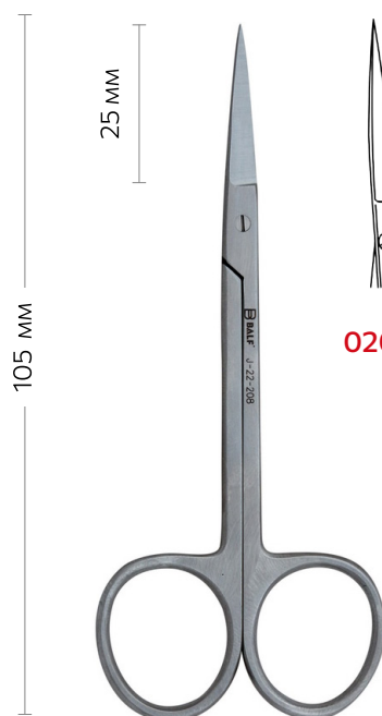
Ножницы хирургические, остроконечные, IRIS
