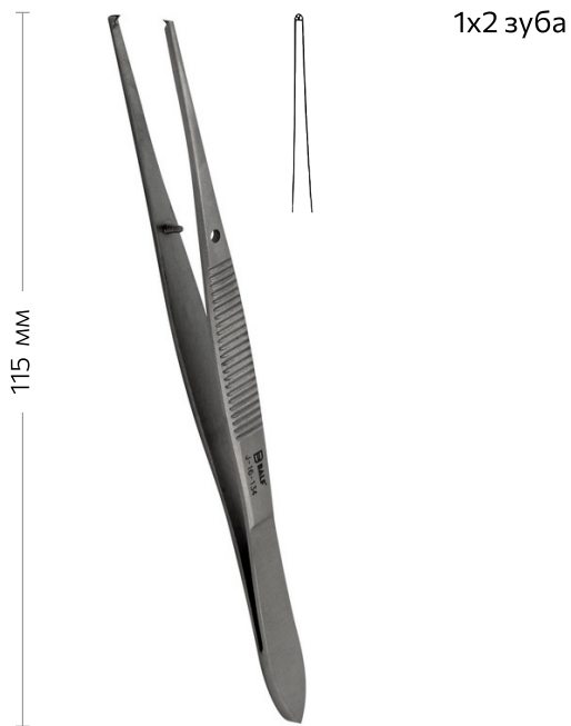
Пинцет хирургический, IRIS
