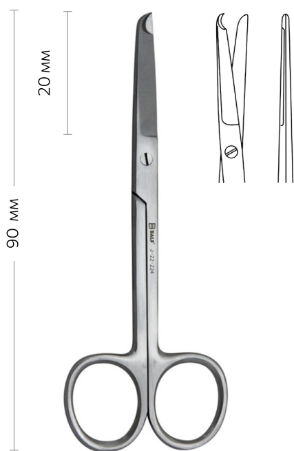
Ножницы для снятия швов, SPENSER
