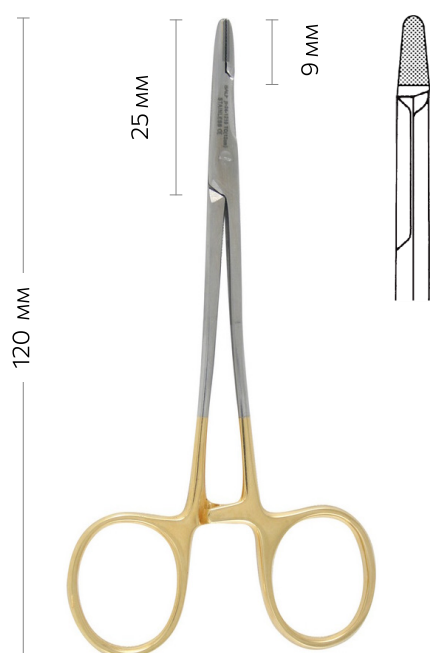
Иглодержатель, N/H, OLSEN HEGAR
