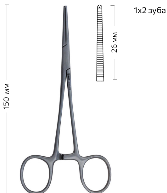
Зажим гемостатический, прямой, LERICHE
